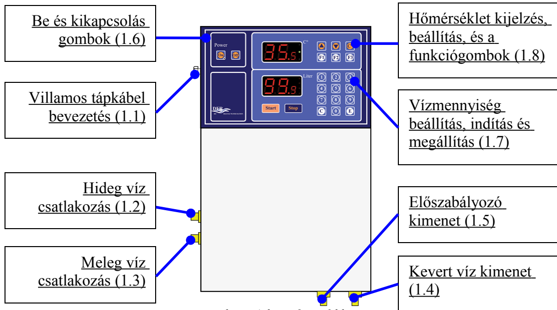
1.1. ábra: A berendezés főbb részei
